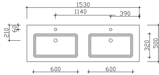
Breite 1530 mm
