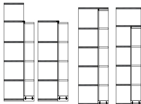
Variante 2 „unter Abdeckblatt / Zwischenbauboden“
