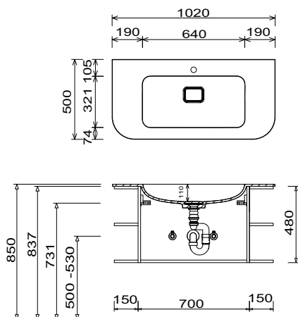
WMS 2610 61 Unterschrankhöhe 480 mm
