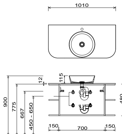
Beispiel Nizza rund Waschtisch Unterschrankhöhe 480 mm
