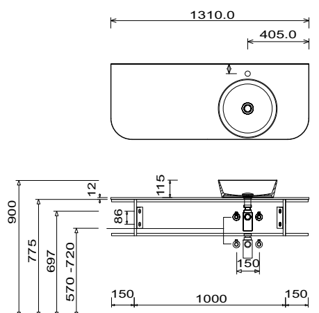
Beispiel Nizza rund Waschtisch Unterschrankhöhe 240 mm
