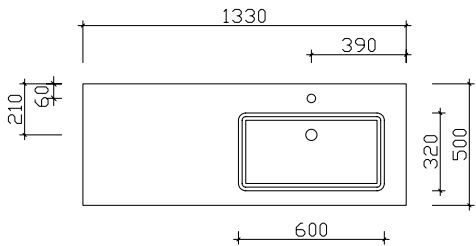
Breite 1330 mm BRE015F13302
