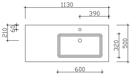
Breite 1130 mm BRE015F11302
