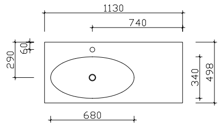
Breite 1130 mm KWT54-1130-L
