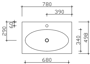
Breite 780 mm KWT54-780
