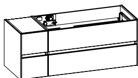
Waschtischunterschrank inkl. LED-Profil mit Bewegungssensor für Griffugen 4 Auszüge, Kosmetikeinsatz im oberen Auszug, 2-teilig
