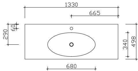
Breite 1330 mm KWT54-1330-M
