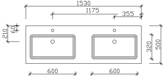
Breite 1530 mm BMD015F15302
