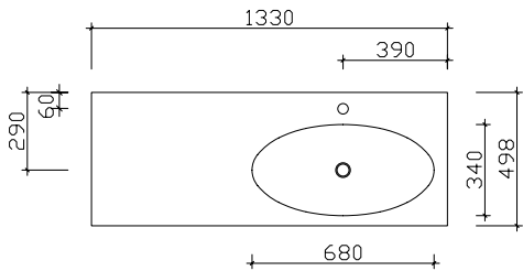
Breite 1330 mm KWT54-1330-R
