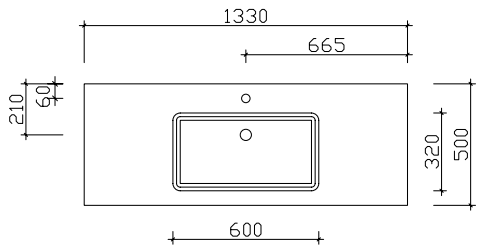
Breite 1330 mm BME015F13302
