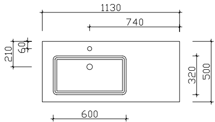
Breite 1130 mm BLE015F11302
