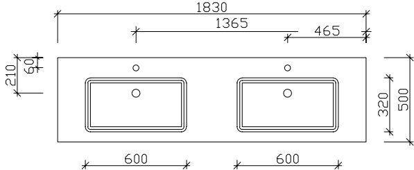
Breite 1830 mm BMD015F18302
