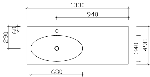
Breite 1330 mm KWT54-1330-L
