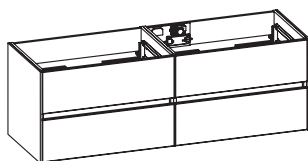
Waschtischunterschrank inkl. LED-Profil mit Bewegungssensor für Grifffugen 4 Auszüge, Kosmetikeinsätze in den oberen Auszügen
