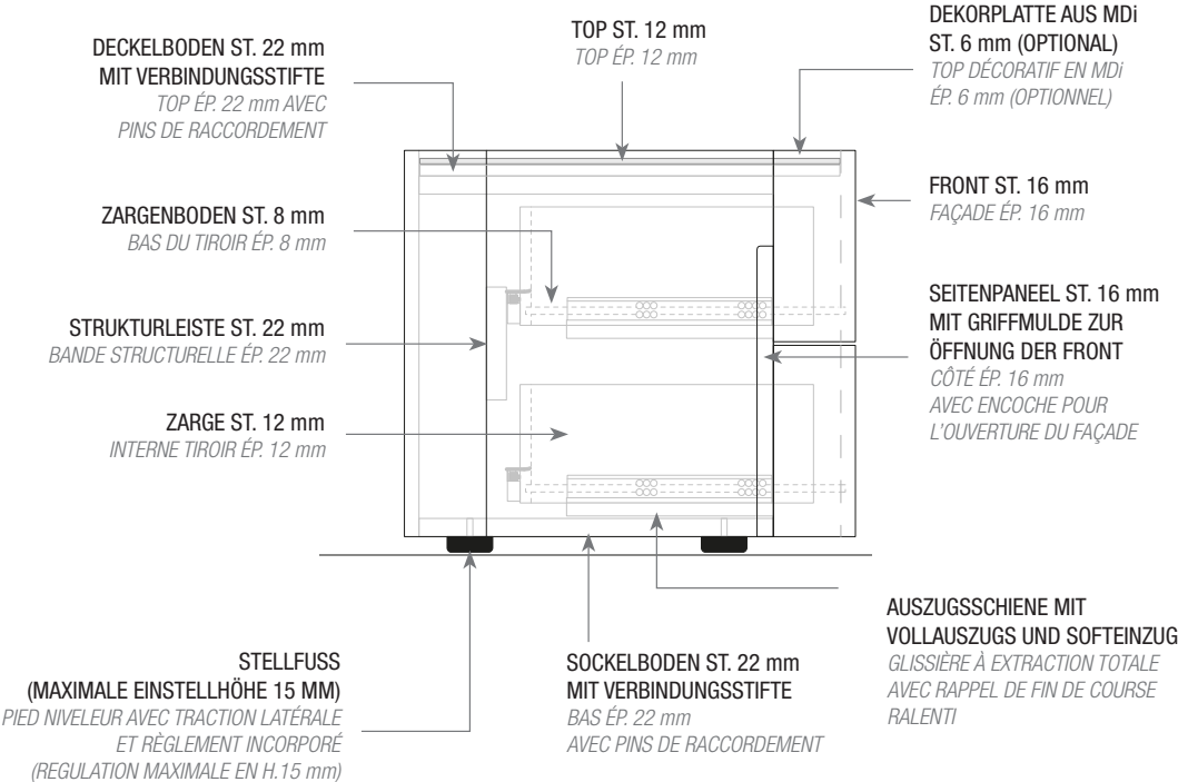
Seitliche sicht vue de côté
