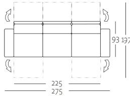
L-SOB-BS mit Funktionsbereich 444/SB225
