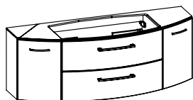
Waschtischunterschrank inkl. LED-Beleuchtung unter dem Waschtisch mit Bewegungssensor 2 Auszüge, 2 Drehtüren, 2 Glaseinlegeböden Sensorschalter (ZCS008E) optional bestellbar zur Steuerung von LEDplus (Farbtemperaturwechsel) bei Waschtischunterschrank!
