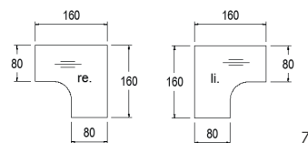
Bsp.-Abb.: C-Fuß
