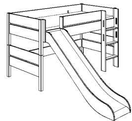
Spielbett mit Rutsche mit Griffleiter, gerade
