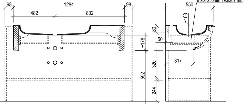
Maßskizze 5
