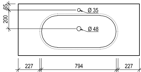
Maßskizze 6
