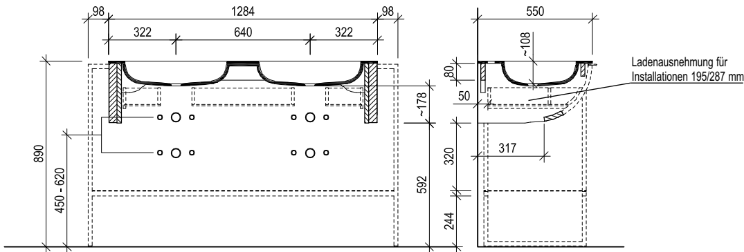
Maßskizze 6
