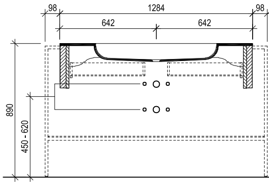
Maßskizze 4
