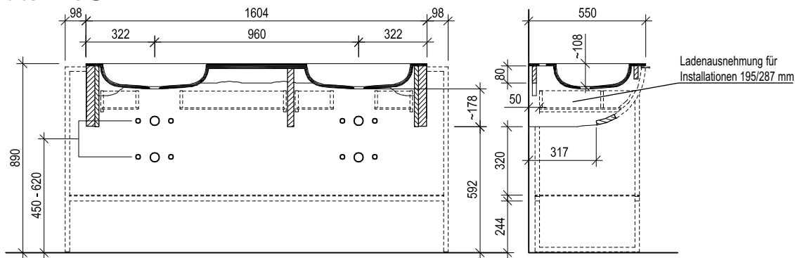
Maßskizze 8
