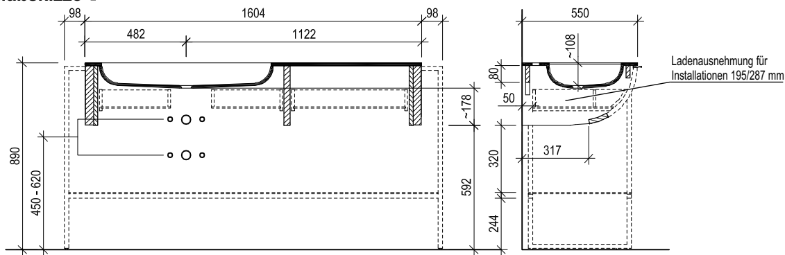
Maßskizze 7
