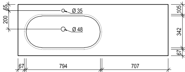
Maßskizze 8
