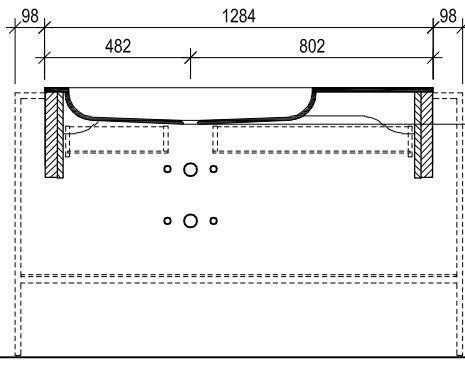
Maßskizze 5
