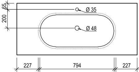
Maßskizze 6
