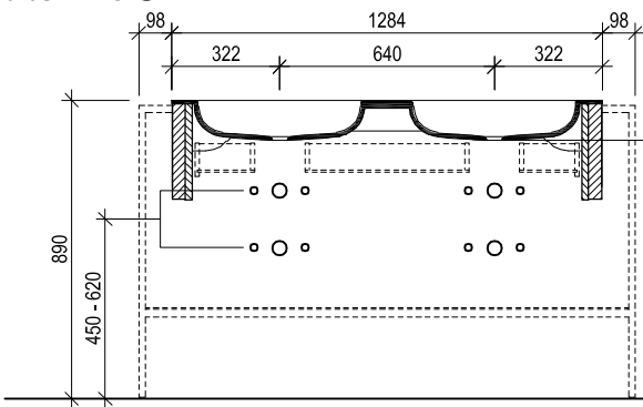
Maßskizze 6
