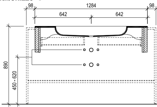
Maßskizze 4
