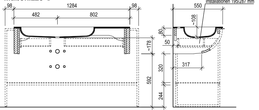
Maßskizze 5
