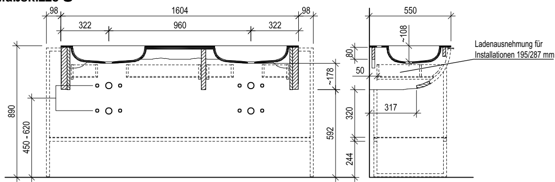
Maßskizze 8
