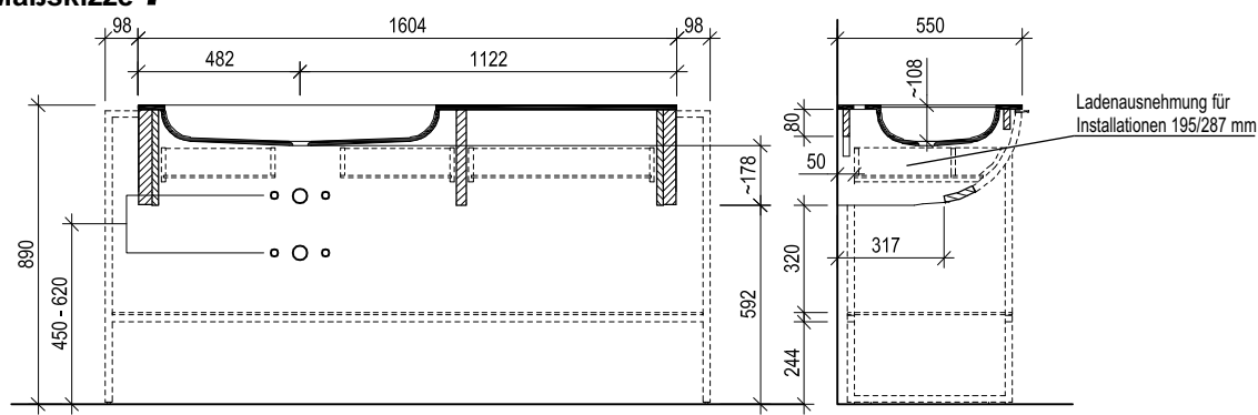
Maßskizze 7
