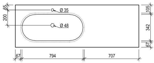
Maßskizze 8
