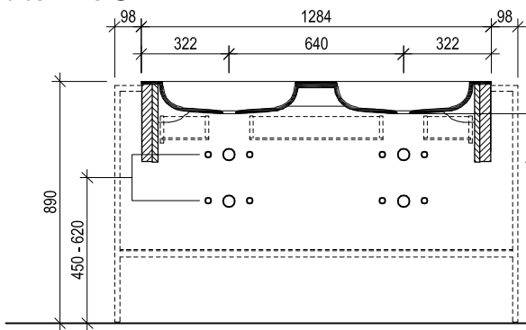
Maßskizze 6
