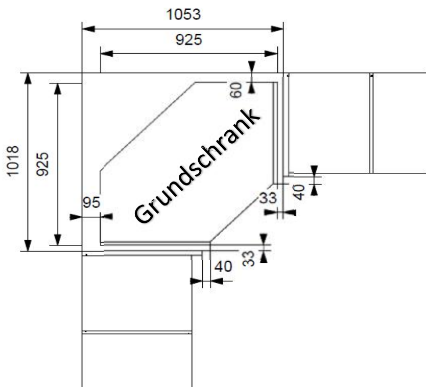
45° Ecke, 1-türig
