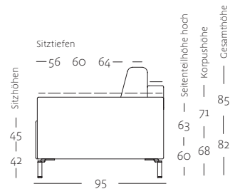
Seitenansicht
