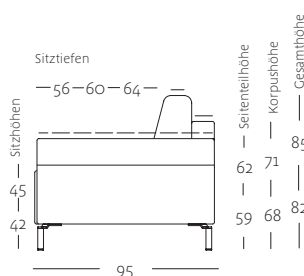
Seitenansicht
