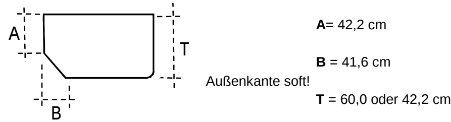
Detail Arbeitsplatte
