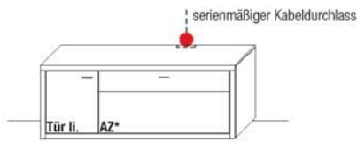
B 148,0 x H 58,0 x T 45,0 cm | AZ* = serienmäßig Vollauszug 1 fester Boden hinter Vollauszug
