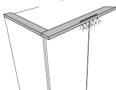
31 Kranz mit Linearbeleuchtung Höhe 3,6 cm Breite 1,4 cm
