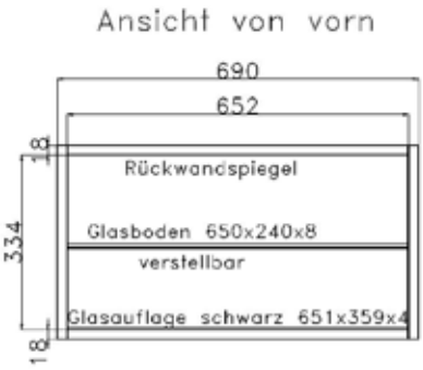
Barfach Korpusbreite 69cm
