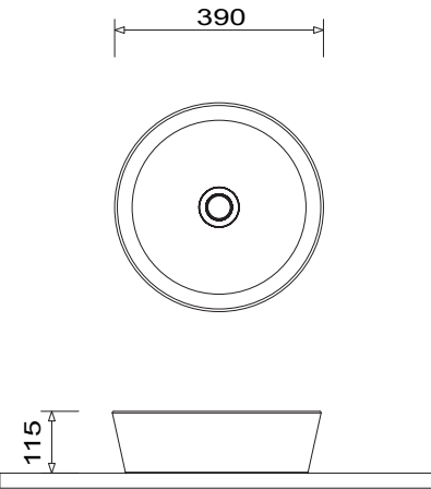
Nizza WTA 3900 1/43 aufgesetzter Waschtisch
