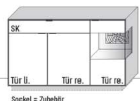
B 151,9 × H 87,9 × T 45,2 cm 3 Böden, 5 Fächer hinter Türen
