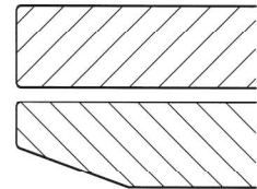
Querschnitt der Tischplatte, MDF 2 x 2,3 cm dick
