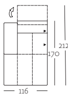
Abschlussessel mit Polstersitz links oder rechts ASS-PSZ 420/116
