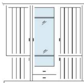
bestehend aus: Regalkorpus 12R 3 x 1272 Tür links 4R 1 x L_F044 Tür rechts 4R 1 x R_F044 Tür links 8R 1 x L_F084 Tür rechts 8R 1 x R_F084 Vitrinentür 10R 1 x R_N104 H/G* Schubkastenpaar 1 x K024
