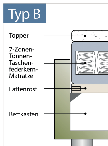
Typ B 7-Zonen-Tonnentaschenfederkern
